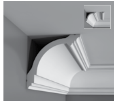
CB512 DUROFOAM® CB512 - 200 x 10 x 10 cm PB513 - 200 x 1,7 x 3,5 cm BXX NEW ∇ = 14,1
