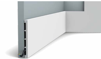
SX168 SQUARE 200 x 15,1 x 1,4 cm Duropolymer®
